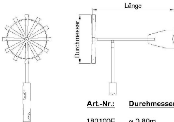
Windrad 12-flüglig
