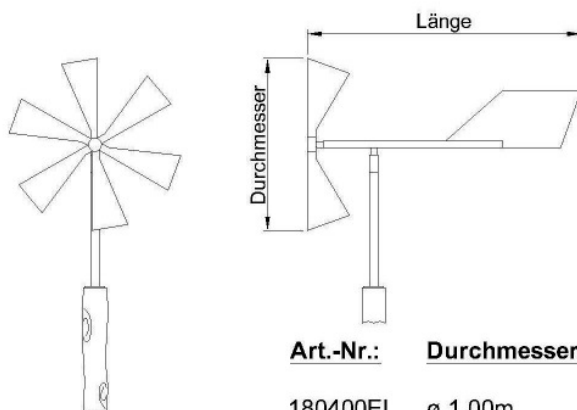
Windrad 6-flüglig
